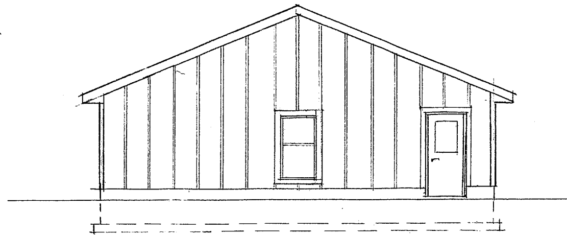
LEFT-SIDE ELEVATION
